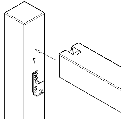
DET 12
