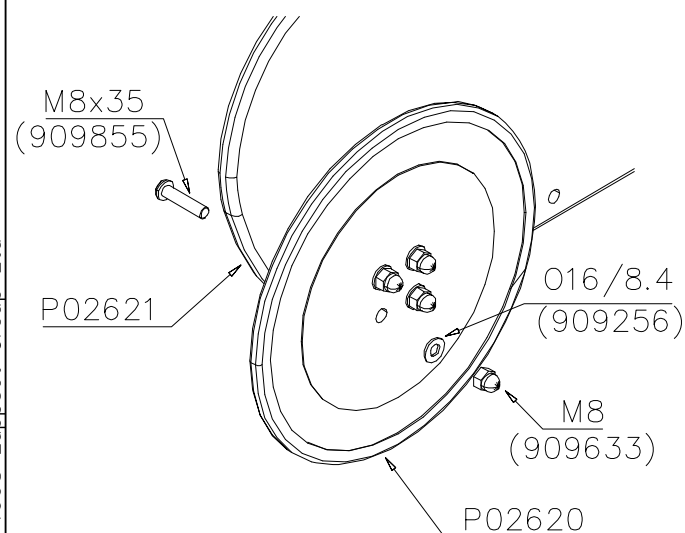
DET 2
