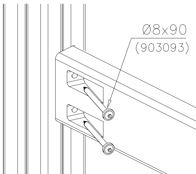
DET 2
