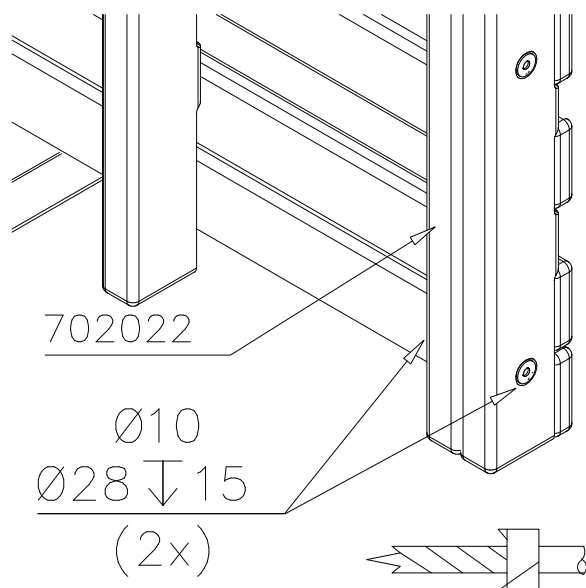
DET 9
