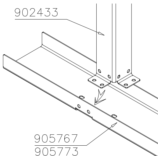
DET 5
