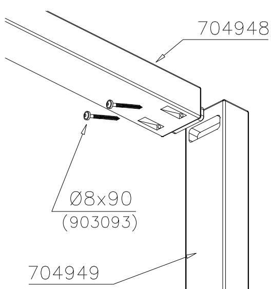
DET 8
