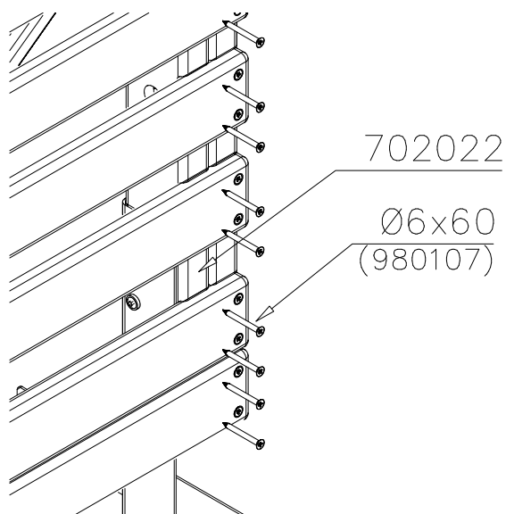
DET 9
