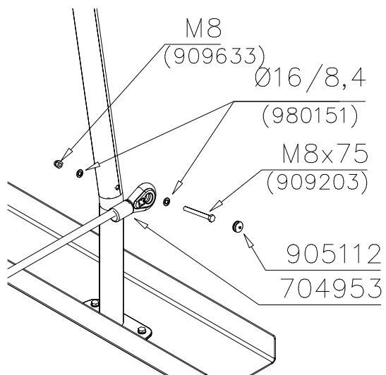
DET 11
