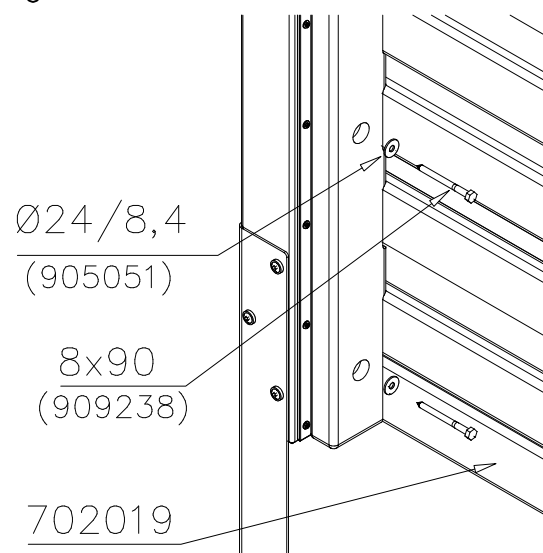
DET 6
