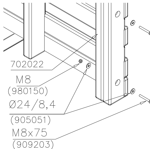
DET 10
