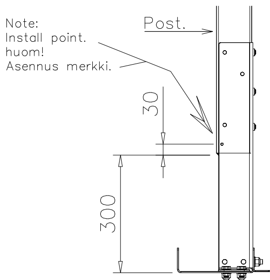
DET 5
