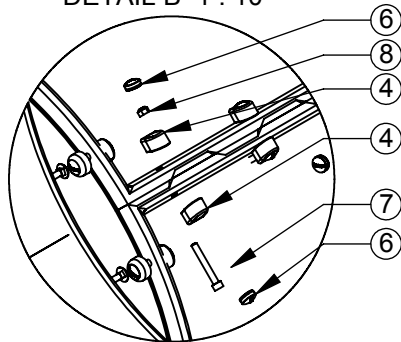
DETAIL B 1 : 10
