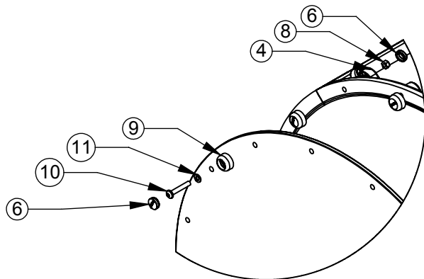
DETAIL C 1 : 10
