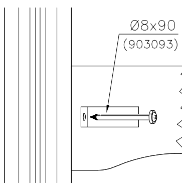
DET 5
