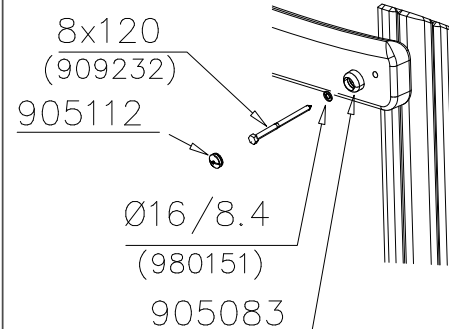
DET 3
