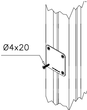
DET 8
