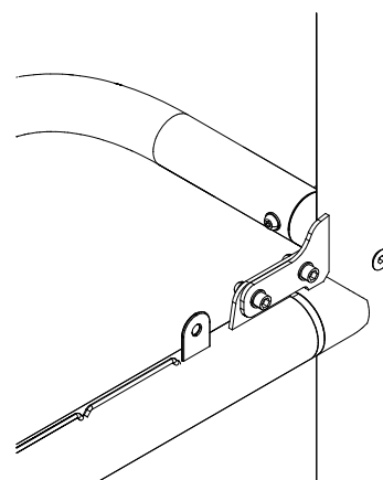
DET 9
