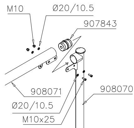
DET 6
