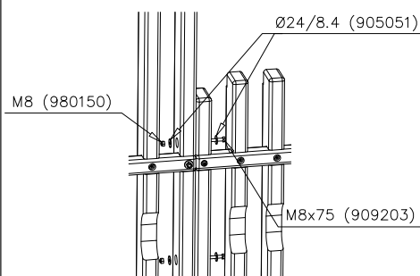
DET 12
