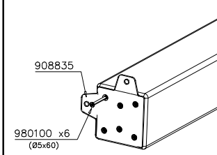
DET 27
