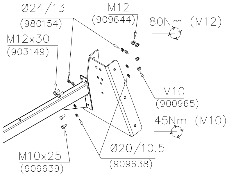
DET A
