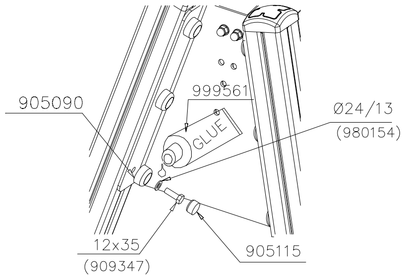
DET B
