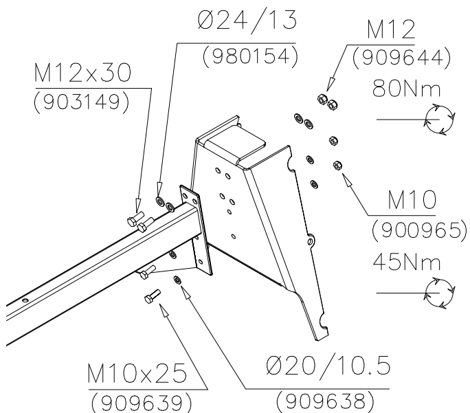
DET B
