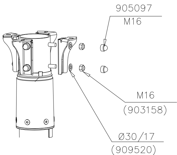
DET 1
