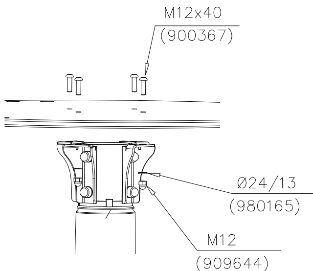
DET 4
