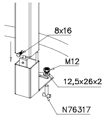
DET 6
