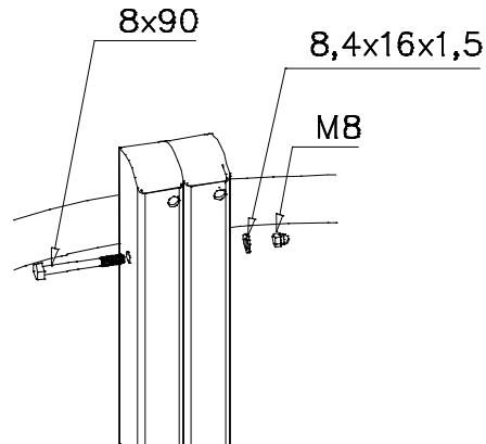
DET 5
