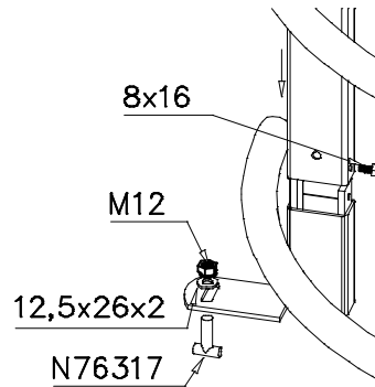
DET 5
