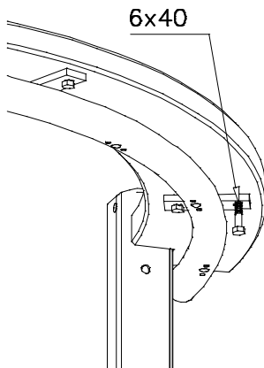
DET 4
