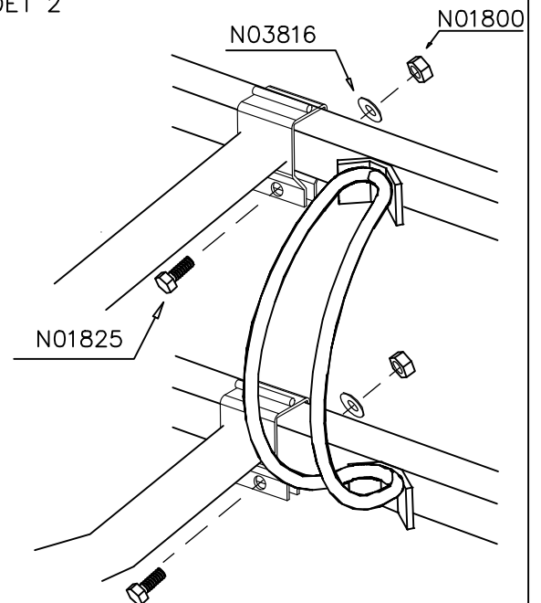
DET 2
