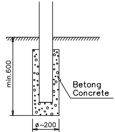
DET 1
