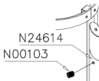
DET 2
