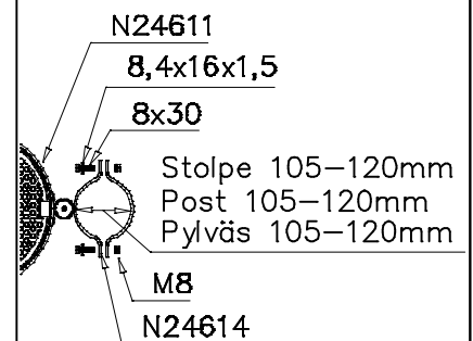
DET 3
