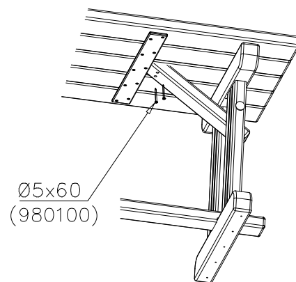
DET 4
