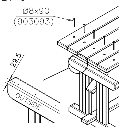
DET 8
