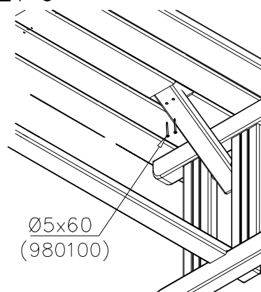
DET 9
