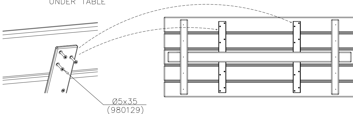
DET 10
