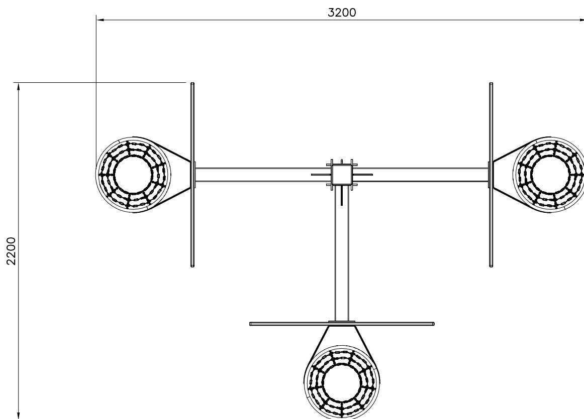
DET 1
