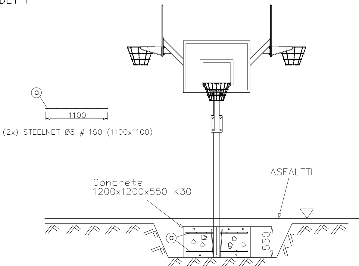
DET 1
