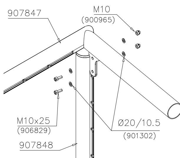
DET 6
