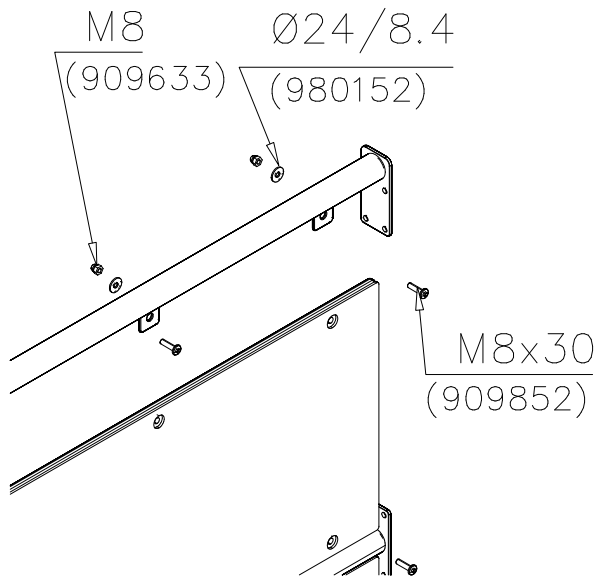
DET 9
