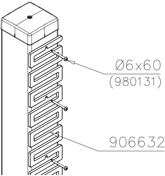
DET 58
