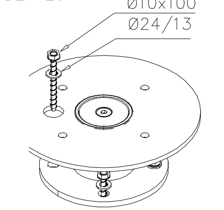
DET 23
