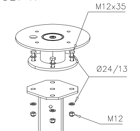
DET 20
