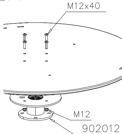
DET 10
