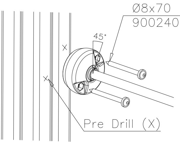
DET 2
