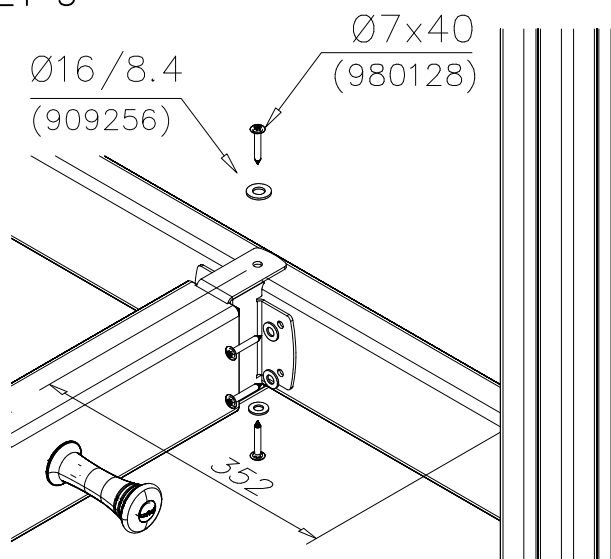
DET 5
