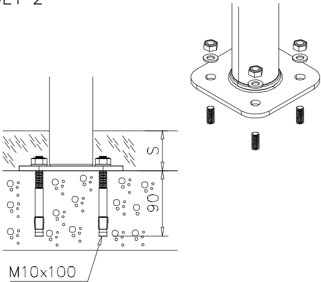
DET 2
