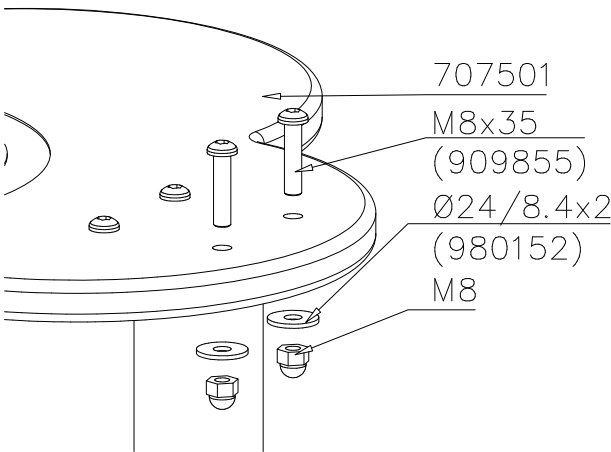
DET 1
