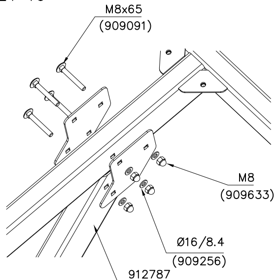
DET 16
