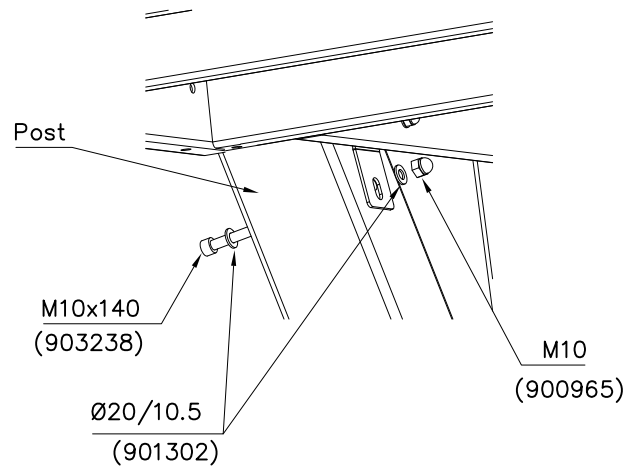
DET 16
