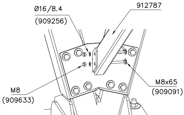
DET 15
