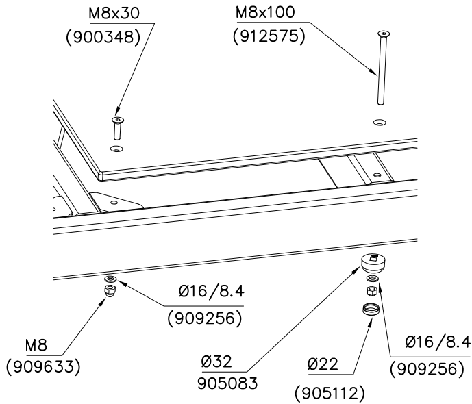
DET 19
