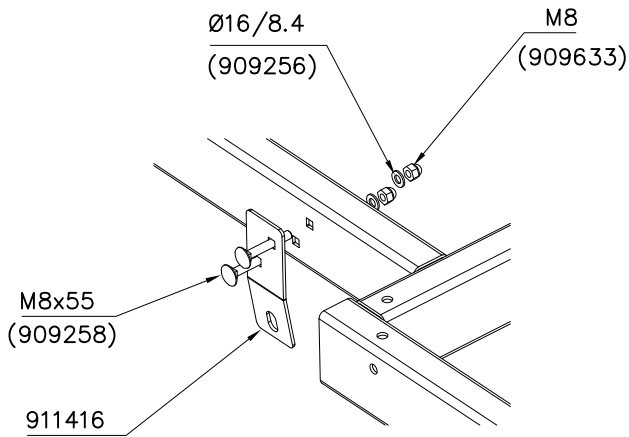
DET 13
