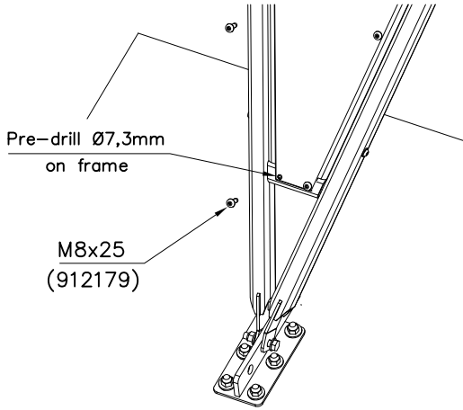
DET 13
