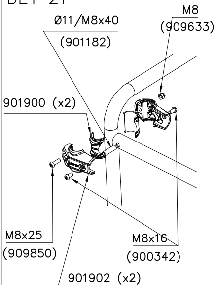
DET 21
