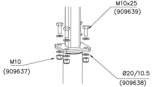
DET 12
