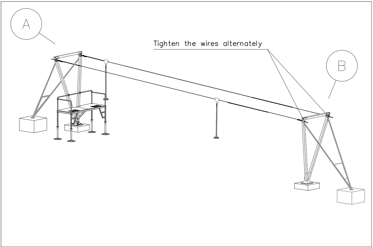
DET 1
