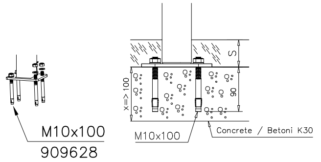
DET 2
