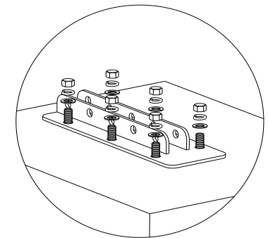
(b) Kiinnityslevy
