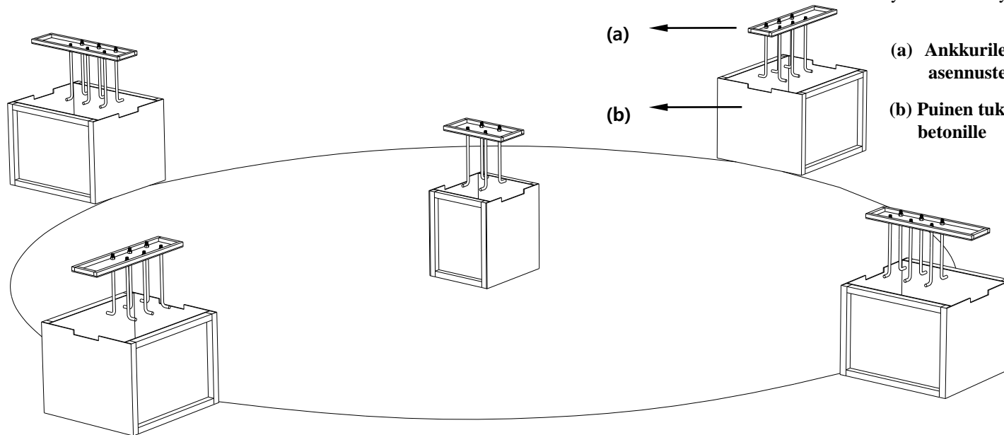
Kuva 6: Puinen tukikehys
