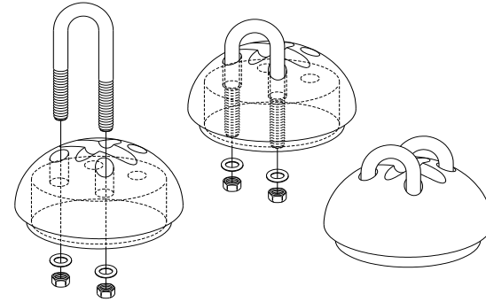
Kuva 14. U-pultin asennus.
