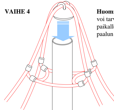
Kuva 15. Paalunkannen asennus.
