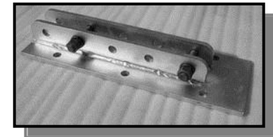
(a) Ankkurilevy
